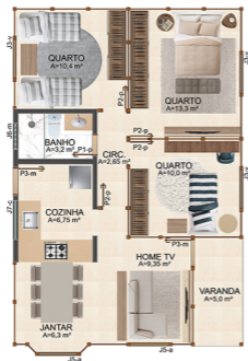
PLANTA TÉRREO
